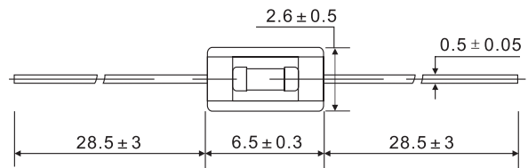
Dimensions(mm)尺寸
