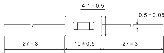
Dimensions(mm)尺寸
